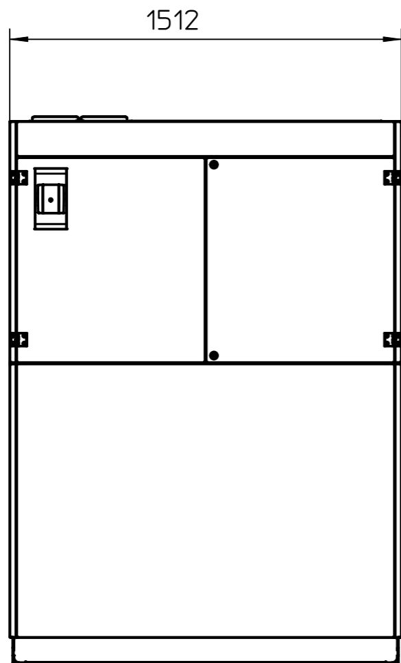
Vorderansicht1
