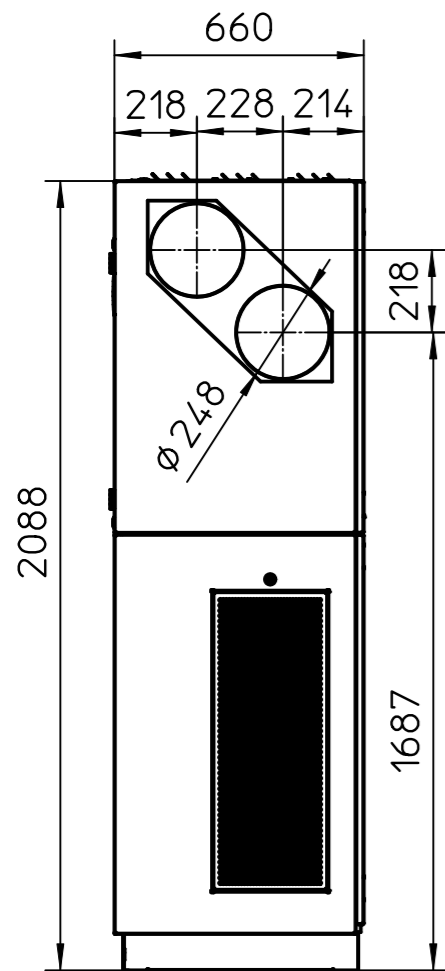
SA rechts1
